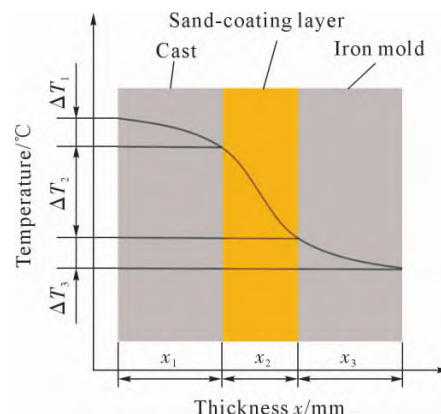
图2 铁型覆砂剖面温度分布
