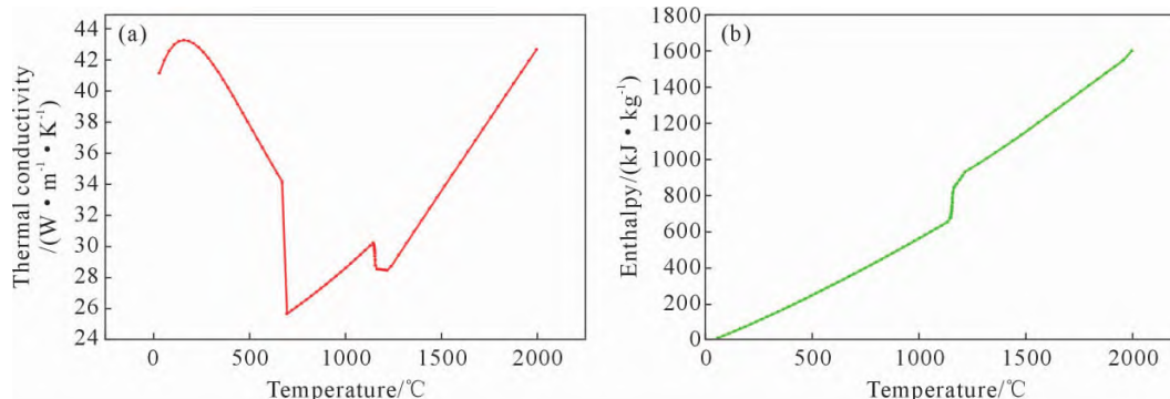
图10 铁型热物性参数:(a)热导率;(b)热焓
