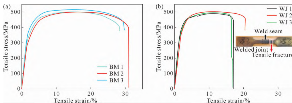
图5 TIG 焊接 Zr-3 母材与接头的拉伸应力-应变曲线:(a) 母材;(b) 焊缝
