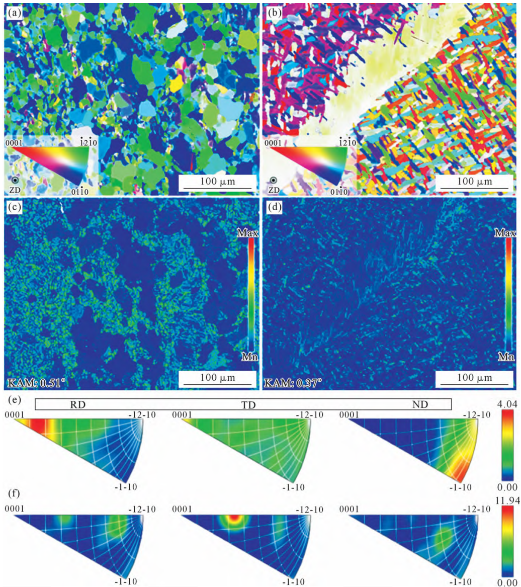
图3 母材与焊缝的IPF、KAM及PF图:(a, c, e)母材;(b, d, f)焊缝
