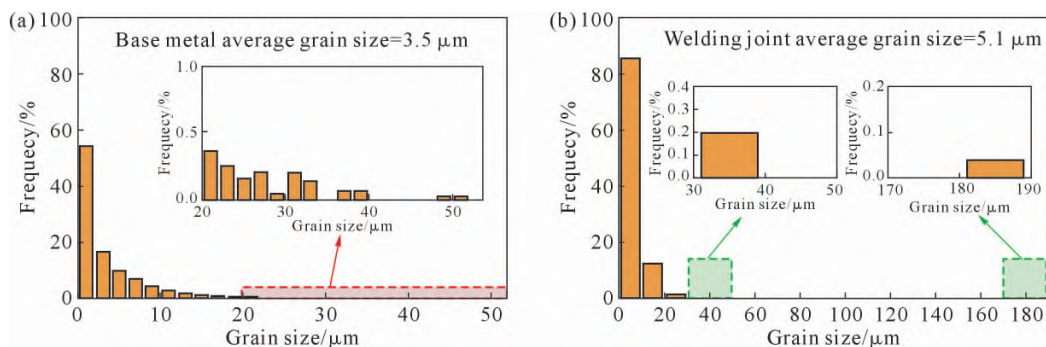
图4 母材与焊缝的晶粒大小尺寸分布:(a)母材;(b)焊缝
