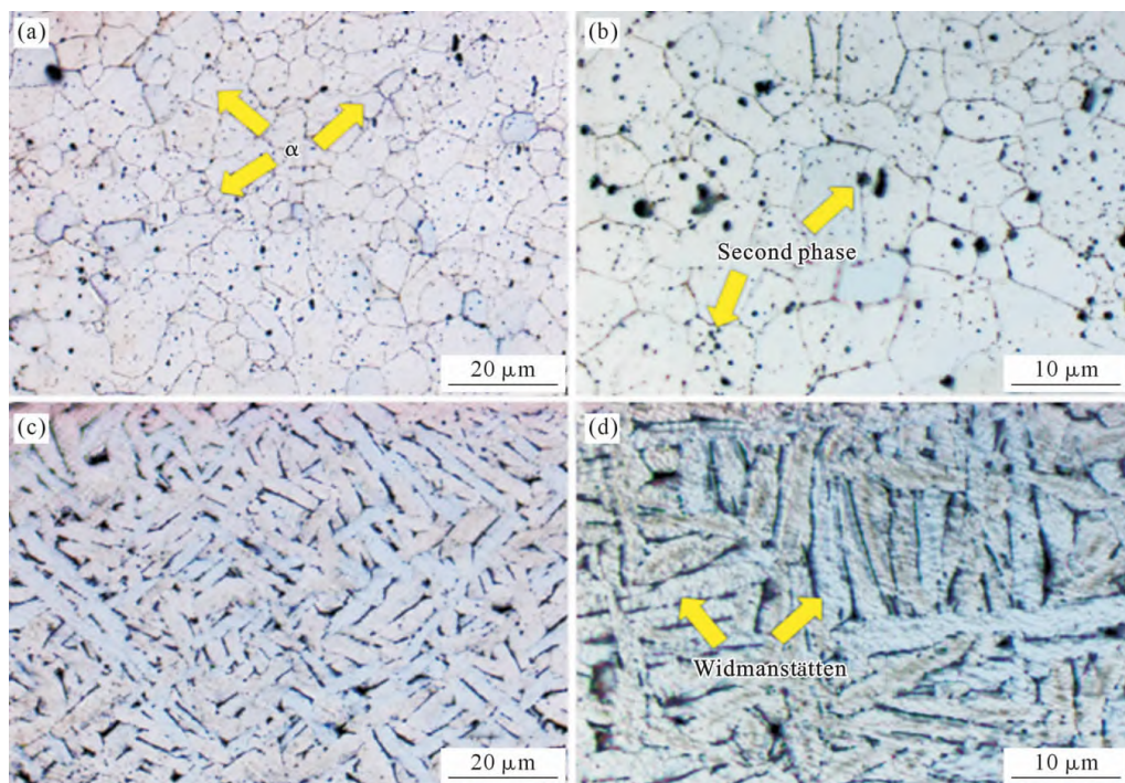
图2 Zr-3 母材与焊缝的显微结构:(a, b) 母材;(c, d) 焊缝
