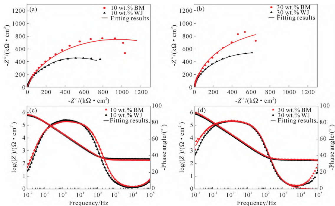
图 8 Zr-3 焊接接头焊缝与母材在不同浓度醋酸溶液中的电化学阻抗谱:(a, b) 焊缝在 10%和 30%浓度下的 bode 图与 Nyquist 图;(c, d) 母材在 10%和 30%浓度下的 bode 图与 Nyquist 图
