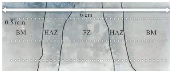
图1 TIG焊接 Zr-3 焊接接头的宏观图
