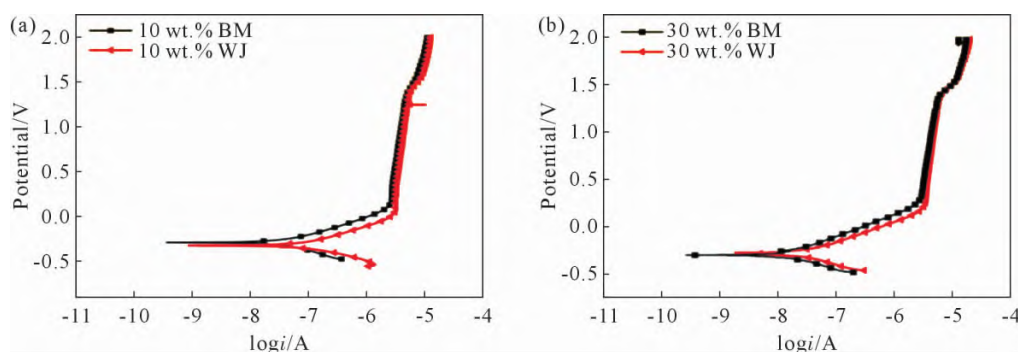
图 9 Zr-3 焊接接头焊缝与母材在不同浓度醋酸溶液中的动电位极化曲线:(a) 10%; (b) 30%
