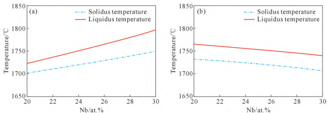
图2 主要元素 Nb 和 Al 对 \text{Ti}_2\text{AlNb} 合金液相线/固相线温度的影响:(a) Ti-22Al-xNb; (b) Ti-25Nb-xAl
