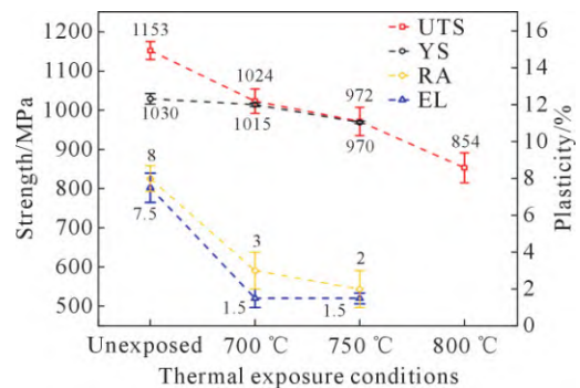
图 6 未暴露与不同温度热暴露试样的室温拉伸性能
