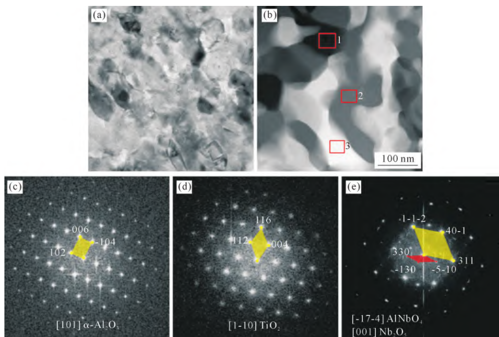
图4 氧化层微观形貌的高角度环形暗场像:(a) 700 °C/50 h;(b) 800 °C/50 h;(c~e) (b) 中1、2、3位置的快速傅里叶变换 Fig.4 High-angle annular dark field images of the oxide layer microstructure: (a) 700 °C/50 h; (b) 800 °C/50 h; (c~e) fast Fourier transforms of positions 1, 2 and 3 in (b)
