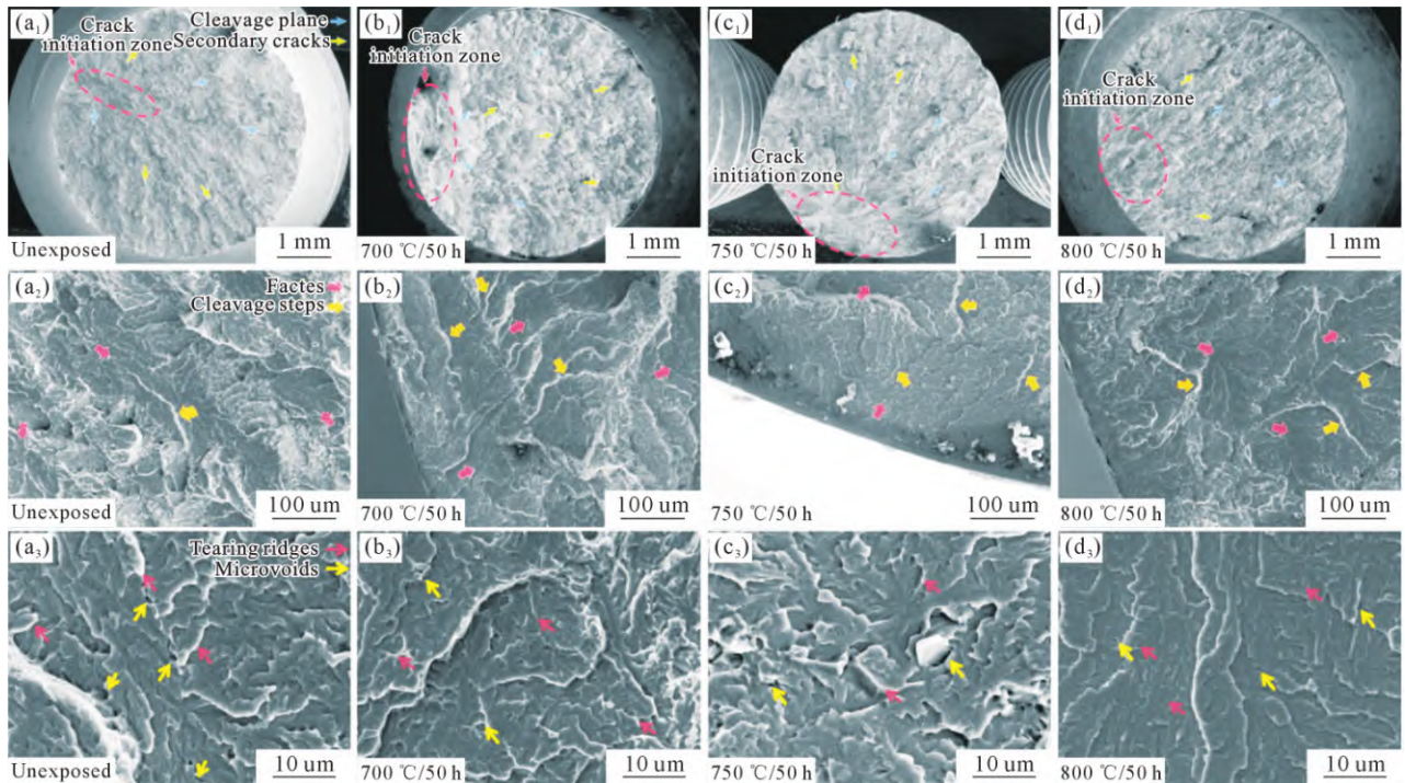
图9 未暴露与不同温度热暴露后宏观及微观断口形貌:(a 1 ~a 3 ) 未暴露;(b 1 ~b 3 ) 700 °C/50 h;(c 1 ~c 3 ) 750 °C/50 h;(d 1 ~d 3 ) 800 °C/50 h
