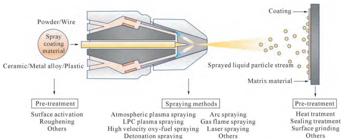
图 3 热喷涂示意图 [107]
