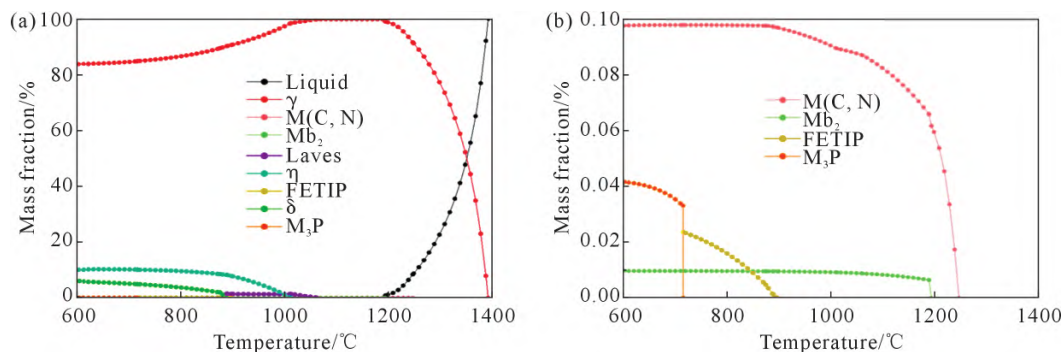
图3 GH4706 合金平衡相图:(a) 性质图;(b) 局部放大图
