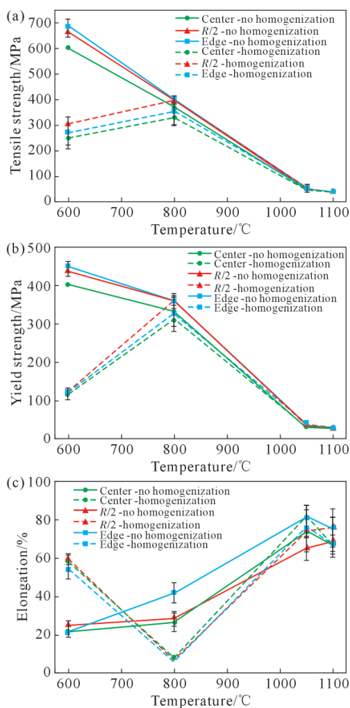
图 10 均匀化处理前后 GH4706 合金的高温拉伸性能对比: (a) 抗拉强度; (b) 屈服强度; (c) 断后伸长率
