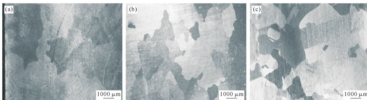
图 9 均匀化处理后 GH4706 合金不同部位的组织形貌:(a) 心部;(b) R/2;(c) 边缘
