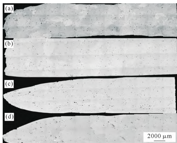
图 11 均匀化后 GH4706 合金 R/2 处在不同拉伸温度下的组织对比: (a) 600 °C; (b) 800 °C; (c) 1 050 °C; (d) 1 100 °C
