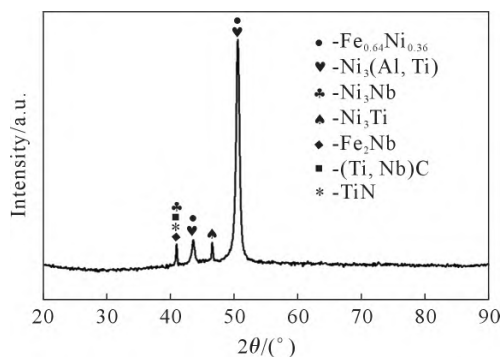
图6 GH4706 合金铸锭的 XRD 谱
