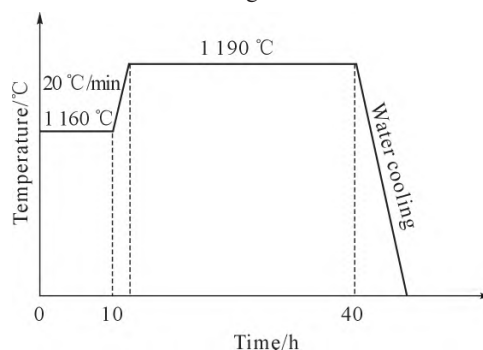
图2 均匀化工艺曲线
