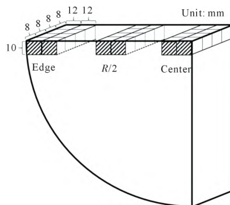
图1 铸锭取样位置示意图
