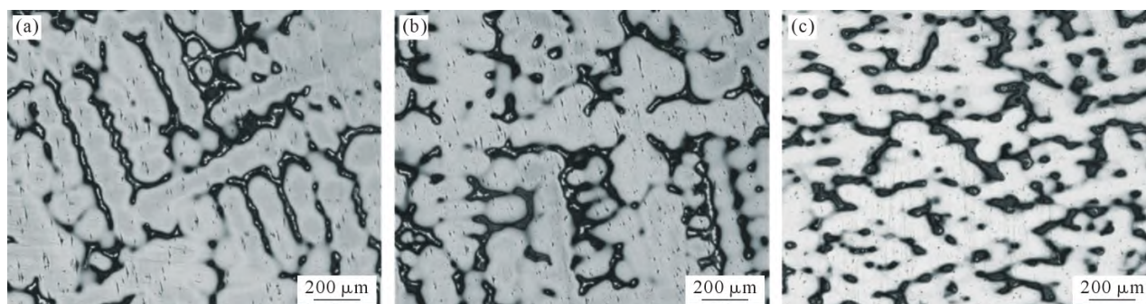
图5 GH4706 合金铸锭不同部位的枝晶形貌:(a) 心部;(b) R/2;(c) 边缘
