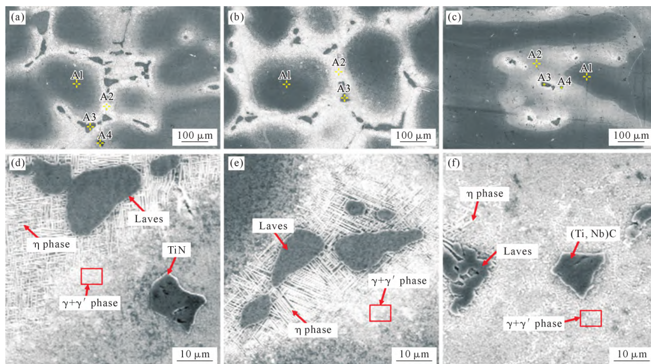
图7 GH4706 合金铸锭不同部位的析出相分布:(a, d) 心部;(b, e) R/2;(c, f) 边缘
