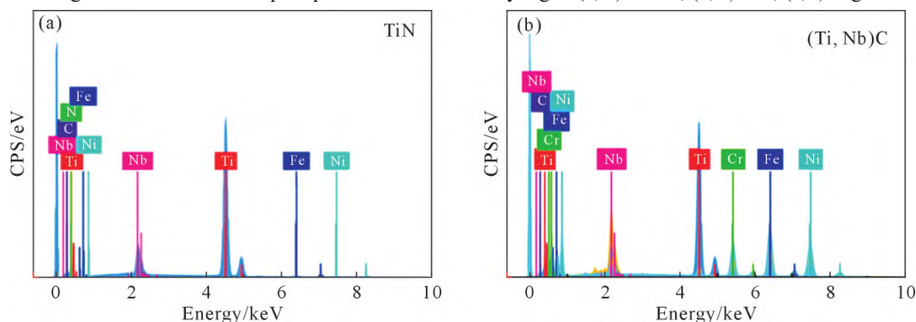
图8 GH4706 合金的 EDS 分析:(a) 图 7a 中 A4;(b) 图 7c 中 A4
