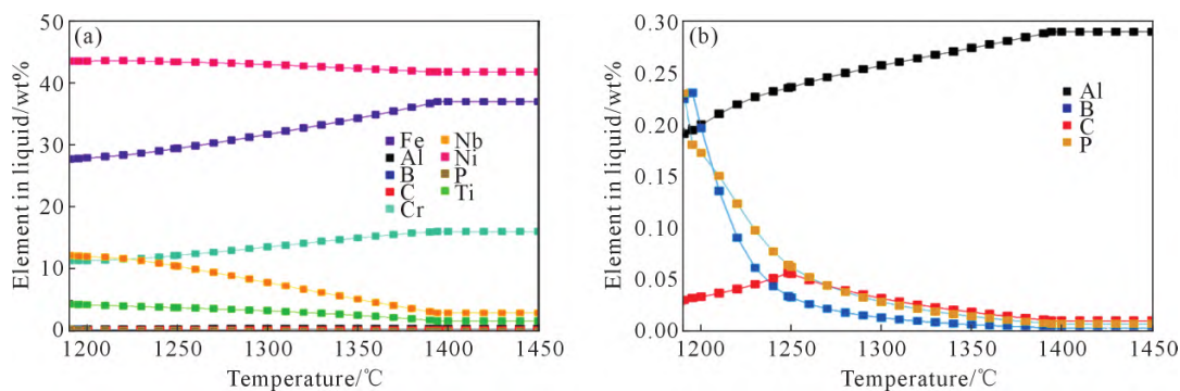
图4 GH4706 合金非平衡凝固过程元素再分配规律:(a) 性质图;(b) Al、B、C、P 局部放大图
