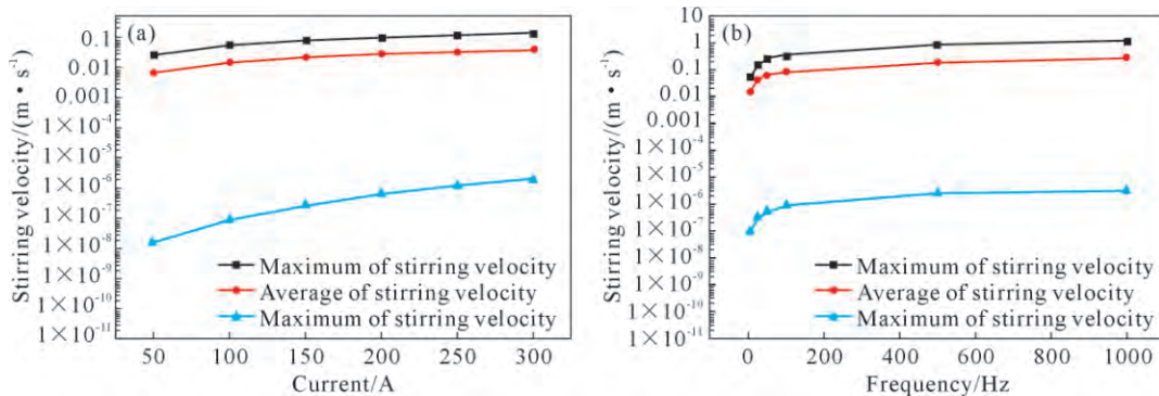
图 13 线圈参数和流场内速度最大值、平均值和最小值的关系:(a) 电流值;(b) 频率
