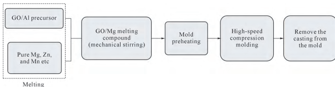
图 2 GO/ZM5 复合材料制备工艺流程
