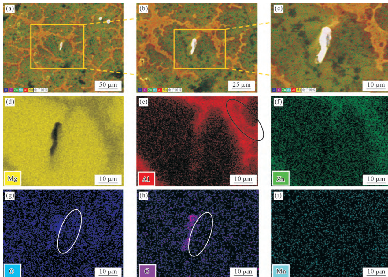
图9 铸态 GO/ZM5 镁基复合材料的 EDS 元素面扫描图;(a~c) EDS 面扫描图;(d~i) Mg、Al、Zn、O、C、Mn 元素分布图
