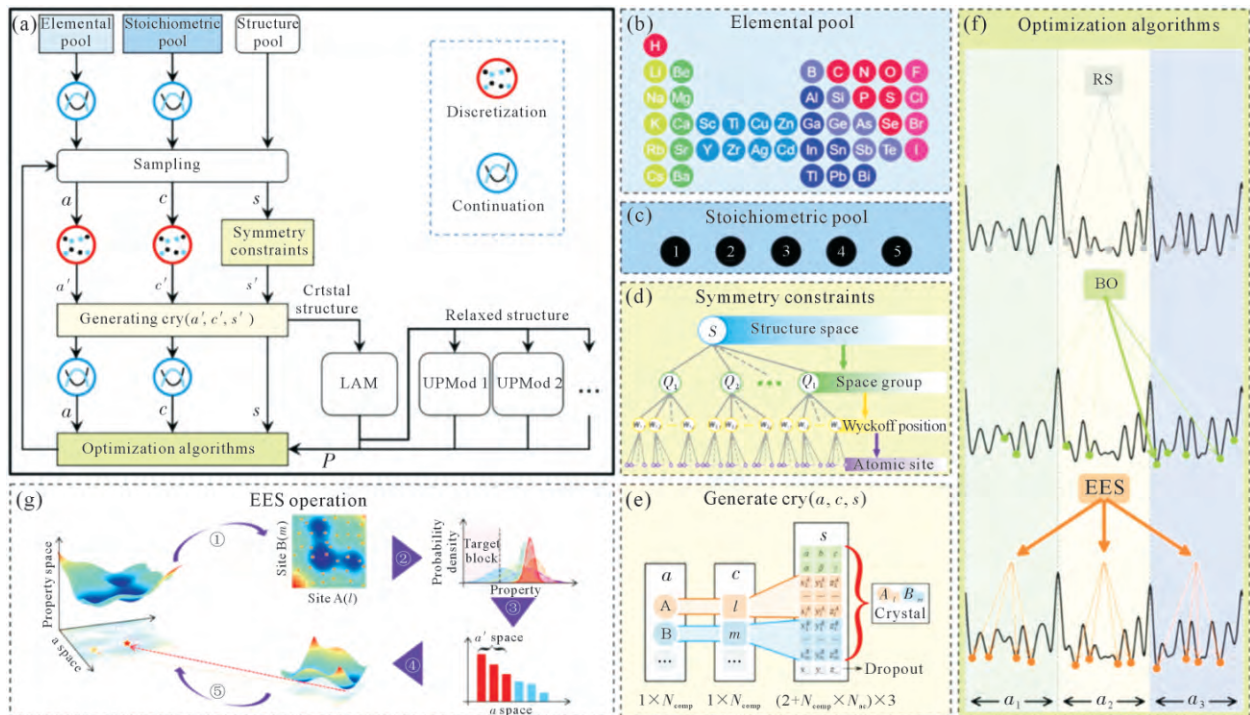
图6 FSIMD 架构:(a) FSIMD 工作流程,主要包括采样生成晶体结构、利用通用机器学习势和通用属性模型进行能量和性质预测以及全空间优化。对 a 和 c 进行离散化和延拓操作,统一生成晶体结构前后的数据类型;(b) 研究过程中使用的 42 种元素;(c) 原子计数池;(d) 生成晶体结构的对称性约束;(e) 晶体数据结构示意图;(f) 随机搜索(RS)、贝叶斯优化(BO)和元素增强采样(EES)探索全空间的性能示意图;(g) EES 操作流程 [63]
