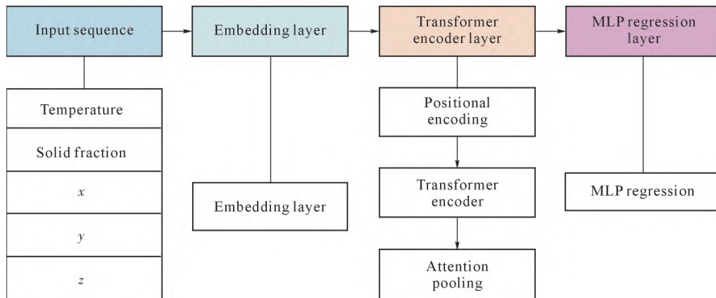
图 5 基于 Transformer 的神经网络回归模型结构示意图
