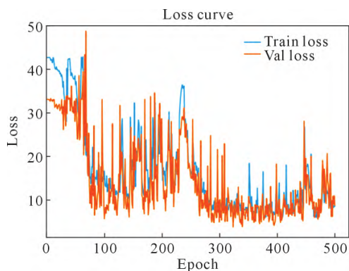
图 8 损失函数曲线 Fig.8 Loss function curves
