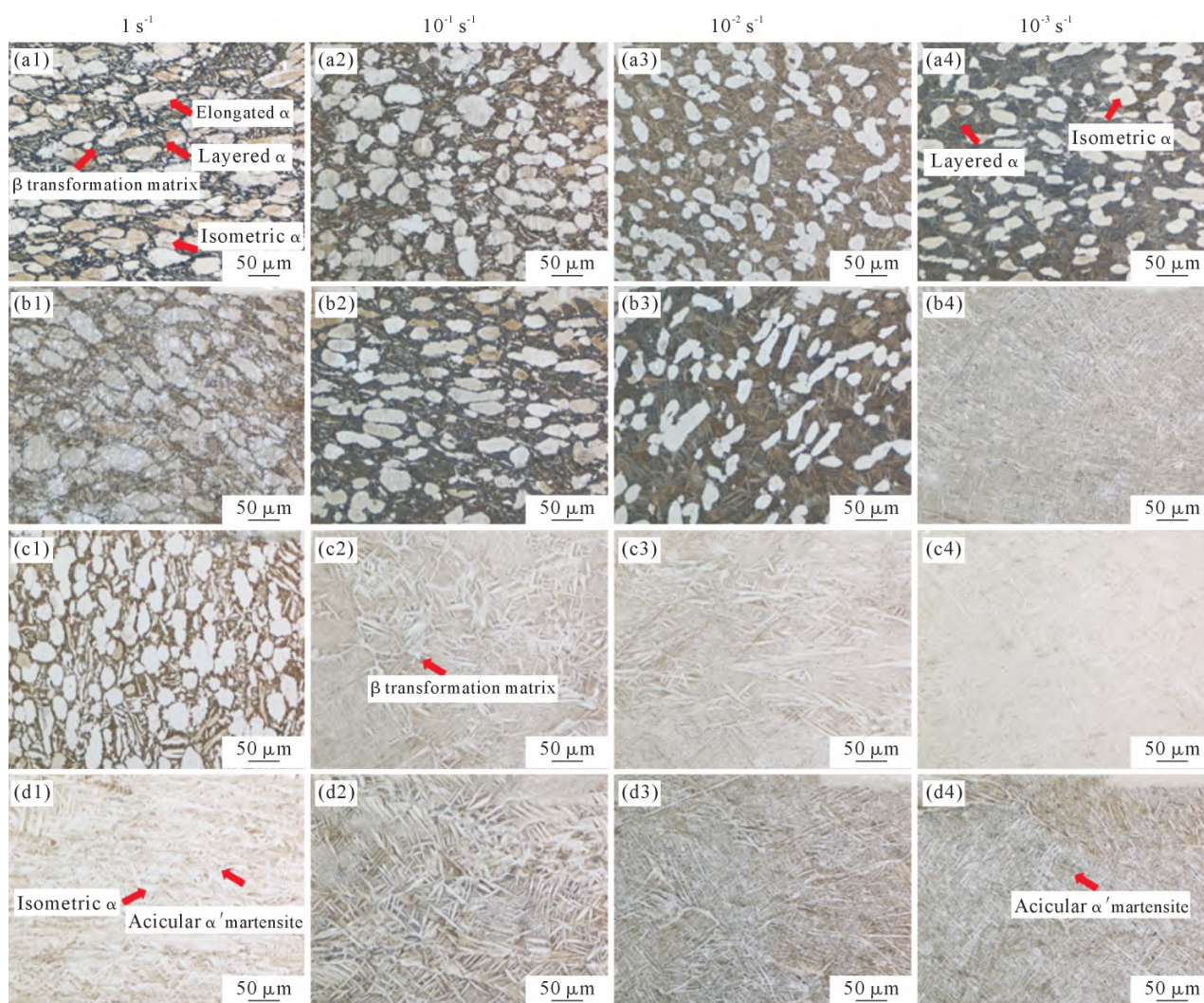
图 11 变形温度与应变速率对 Ti150 钛合金显微组织的影响: (a1~a4) 970 °C; (b1~b4) 1 000 °C; (c1~c4) 1 020 °C; (d1~d4) 1 040 °C
