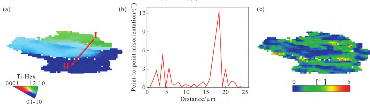
图 14 变形温度 1 000 °C、应变速率 1 s -1 下 α 晶粒内的显微组织表征结果:(a) IPF 图;(b) 晶粒内点到点取向差;(c) 晶粒内的 KAM
