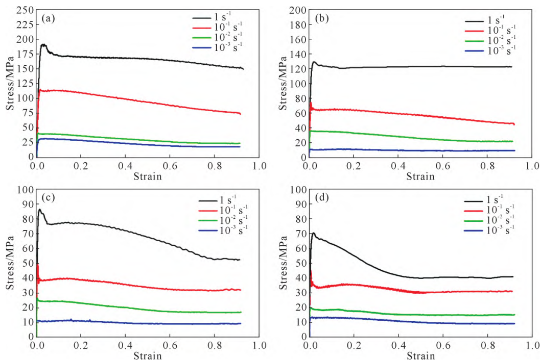
图3 Ti150 钛合金不同条件下的应力-应变曲线:(a) 970\text{ }^\circ\text{C} ; (b) 1\text{ }000\text{ }^\circ\text{C} ; (c) 1\text{ }020\text{ }^\circ\text{C} ; (d) 1\text{ }040\text{ }^\circ\text{C}
