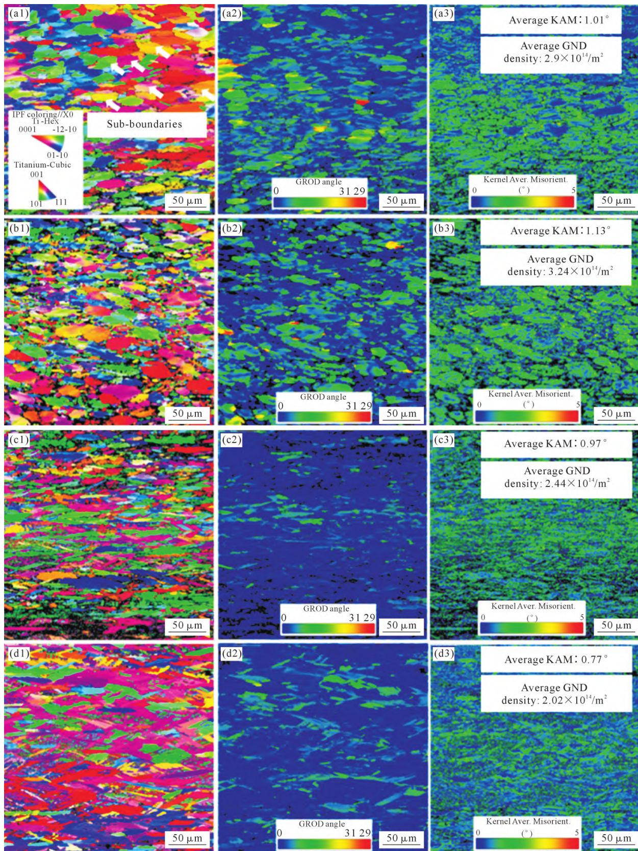
图 12 变形温度 1 000 °C 下不同应变速率对 Ti150 钛合金显微组织表征结果:(a1~a3) 应变速率 1 \text{ s}^{-1} 下 IPF、GROD 和 KAM 图;(b1~b3) 应变速率 10^{-1} \text{ s}^{-1} 下 IPF、GROD 和 KAM 图;(c1~c3) 应变速率 10^{-2} \text{ s}^{-1} 下 IPF、GROD 和 KAM 图;(d1~d3) 应变速率 10^{-3} \text{ s}^{-1} 下 IPF、GROD 和 KAM 图
