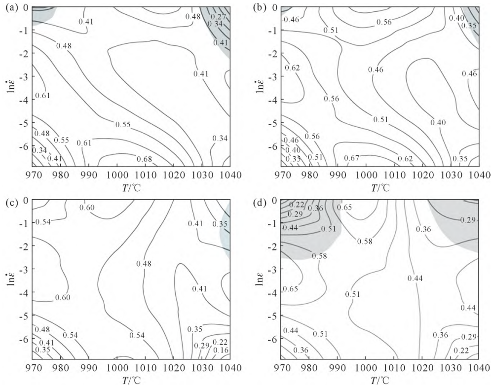
图 10 不同应变量下的热加工图: (a) \varepsilon=0.2 ; (b) \varepsilon=0.4 ; (c) \varepsilon=0.6 ; (d) \varepsilon=0.8
