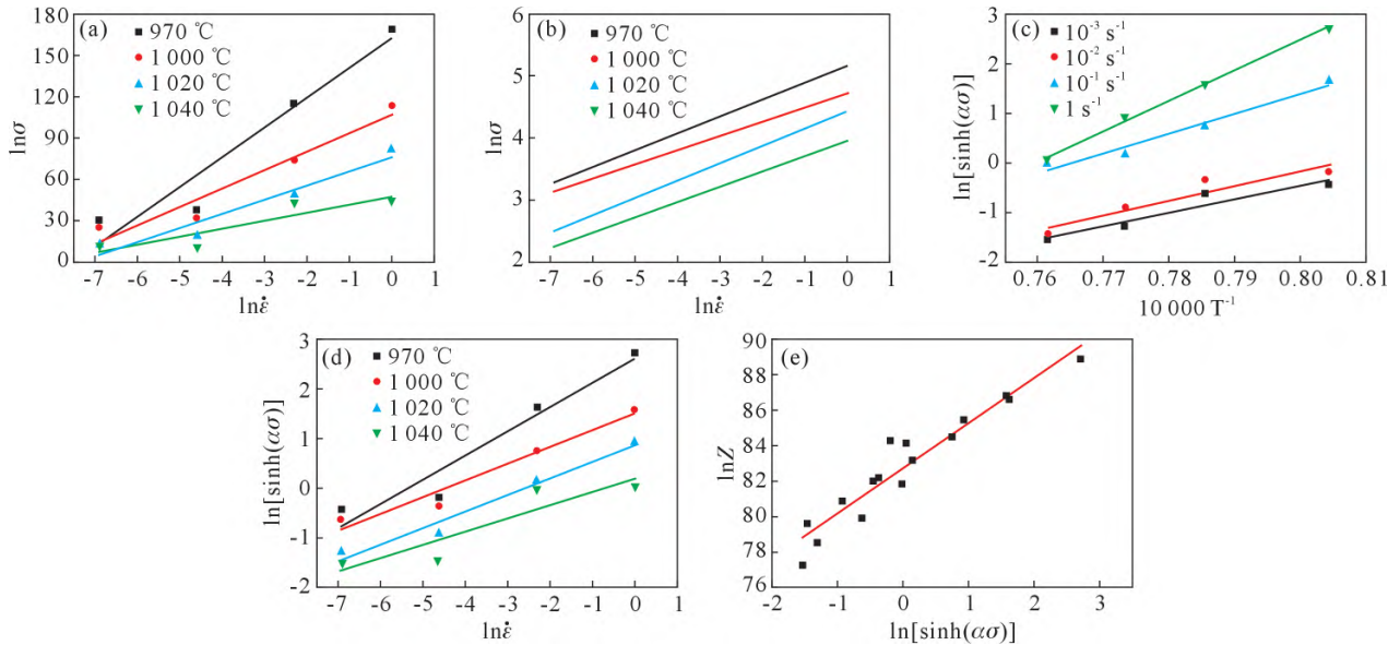
图7 Ti150 钛合金的线性拟合结果:(a) \sigma - \ln\dot{\epsilon} ; (b) \ln\sigma - \ln\dot{\epsilon} ; (c) \ln[\sinh(\alpha\sigma)] - 10000/T ; (d) \ln[\sinh(\alpha\sigma)] - \ln\dot{\epsilon} ; (e) \ln Z - \ln[\sinh(\alpha\sigma)]
