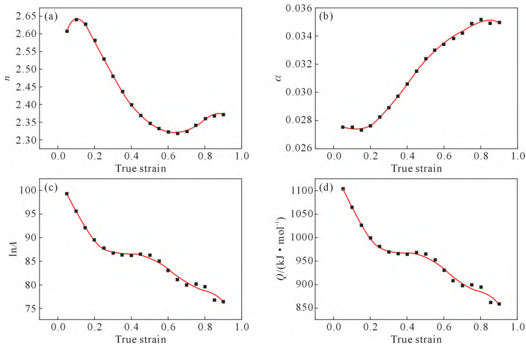
图8 Ti150 钛合金不同应变下材料常数的多项式拟合:(a) n ; (b) \alpha ; (c) \ln A ; (d) Q
