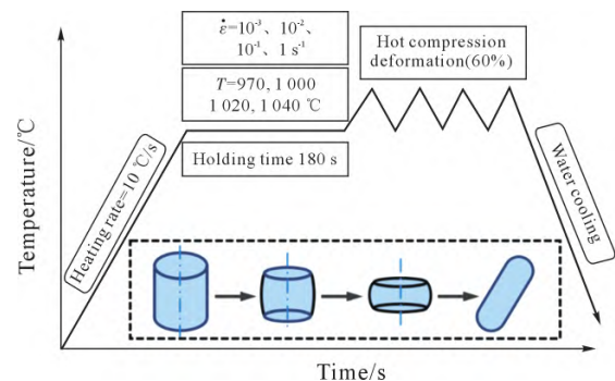
图 2 热压缩试验过程示意图 Fig.2 Schematic diagram of the thermal compression test process
