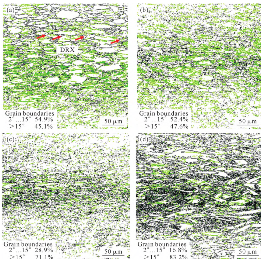
图 13 变形温度 1 000 °C 下不同应变速率的晶界分布图:(a) 1 s -1 ; (b) 10 -1 s -1 ; (c) 10 -2 s -1 ; (d) 10 -3 s -1 Fig.13 Grain boundary distribution maps at a deformation temperature of 1 000 °C under different strain rates: (a) 1 s -1 ; (b) 10 -1 s -1 ; (c) 10 -2 s -1 ; (d) 10 -3 s -1
