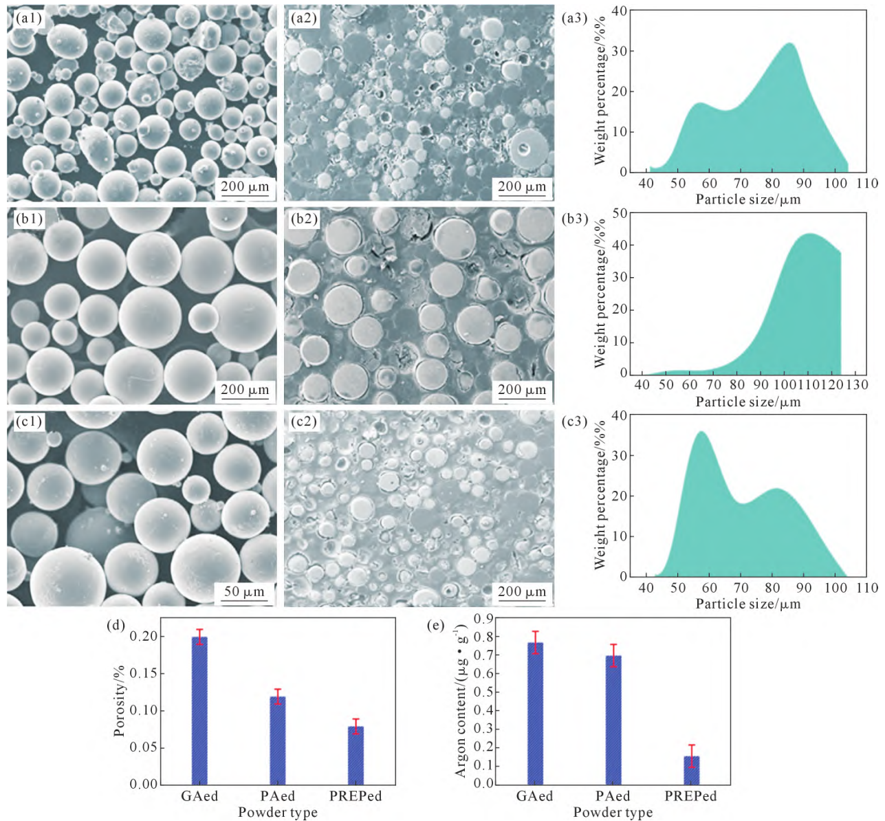
图4 不同工艺制备 Ti6Al4V 粉末的微观组织与性能:(a1, b1, c1) GA、PREP 和 PA 制备的 Ti6Al4V 粉末表面微观组织;(a2, b2, c2) GA、PREP 和 PA 制备的 Ti6Al4V 粉末截面微观组织;(a3, b3, c3) GA、PREP 和 PA 制备的 Ti6Al4V 粉末粒度分布;(d, e) 粒径 150 \mu\text{m} 以下雾化粉末孔隙率和氩含量 [45]
