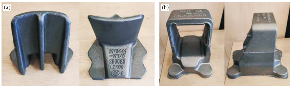
图 9 ADI1050-6 满足长春一汽某新能源卡车的要求:(a) 前支架-辅助钢板弹簧;(b) 后平衡悬架板簧左支座-中桥左侧(吉林省博铤机械制造有限公司提供)
