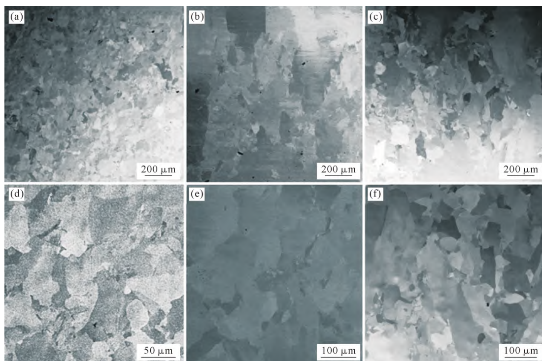
图5 激光定向能量沉积 Ti-6Al 合金样品 XOY 、 XOZ 、 YOZ 面的 EBSD: (a, d) XOY 面; (b, e) XOZ 面; (c, f) YOZ 面 Fig.5 EBSD in the XOY , XOZ and YOZ planes of the LDED Ti-6Al alloys: (a, d) XOY plane; (b, e) XOZ plane; (c, f) YOZ plane
