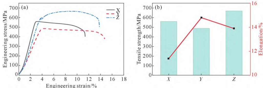
图8 激光定向能量沉积 Ti-6Al 合金分别沿 X、Y、Z 方向的拉伸性能:(a) 工程应力-应变曲线;(b) 性能统计
