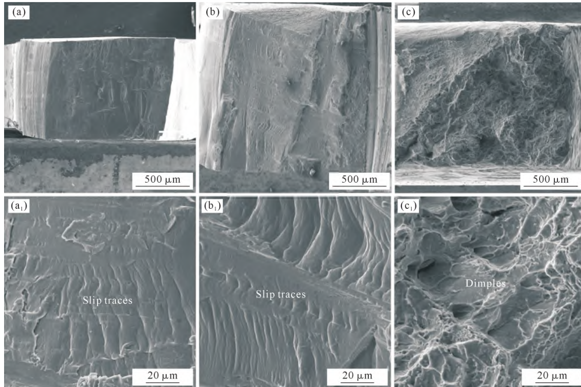
图 10 激光定向能量沉积 Ti-6Al 合金分别沿 X 、 Y 、 Z 方向拉伸断口形貌:(a, a 1 ) X 方向;(b, b 1 ) Y 方向;(c, c 1 ) Z 方向 Fig.10 Tensile fracture morphology of the LDED Ti-6Al alloy along the X , Y and Z directions: (a, a 1 ) X direction; (b, b 1 ) Y direction; (c, c 1 ) Z direction
