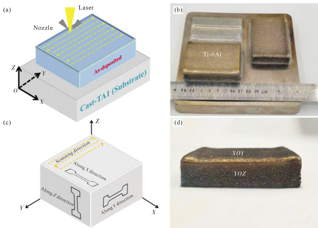
图2 LDDED 成形示意图与 Ti-6Al 合金块体实物:(a) 成形示意图;(b) 取样示意图;(c, d) Ti-6Al 合金块体实物
