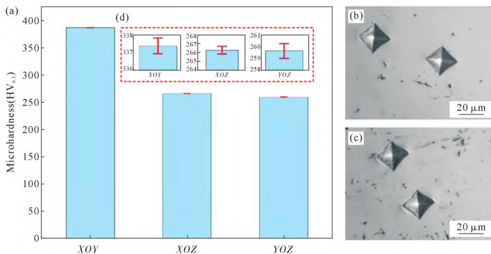
图9 激光定向能量沉积 Ti-6Al 合金样品 XOY、XOZ、YOZ 面的显微硬度:(a, d) 显微硬度及局部放大图;(b, c) XOZ、YOZ 面硬度压痕
