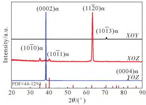
图3 激光定向能量沉积 Ti-6Al 合金 XRD 图谱 Fig.3 XRD patterns of the LDED Ti-6Al alloy
