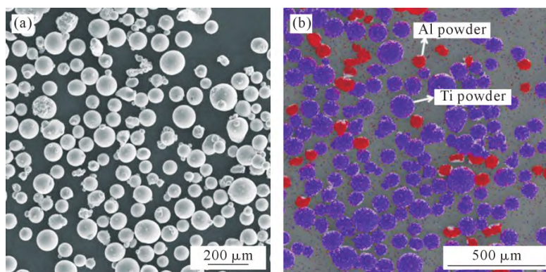
图1 Ti-6Al 混合粉末形貌与 EDS 面扫:(a) SEM 图;(b) EDS 面扫
