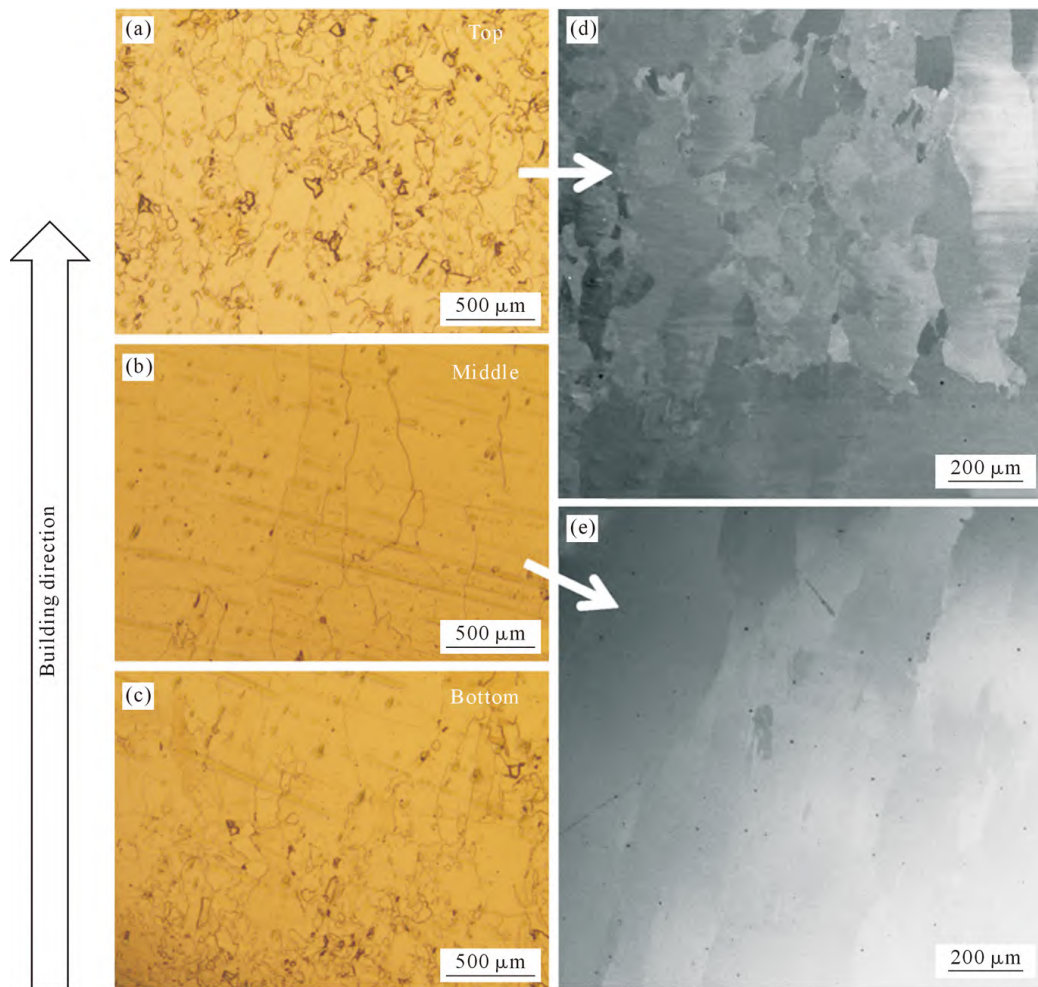
图4 激光定向能量沉积 Ti-6Al 合金样品 XOZ 面微观形貌:(a~c) 沿建造方向 XOZ 面顶部、中部、底部的腐蚀金相;(d, e) XOZ 面顶部及中部对应 SEM 图像
