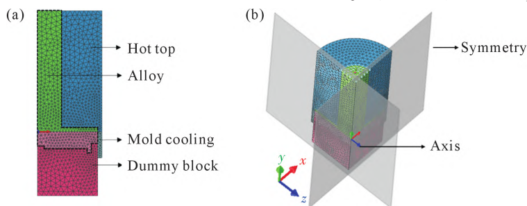
图4 几何模型的网格划分 Fig.4 Geometric meshing
