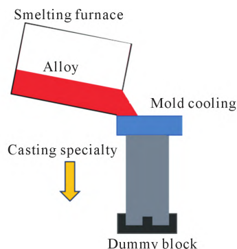
图 1 2024 铝合金半连铸工艺流程
