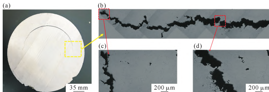
图3 环状裂纹:(a) 环状裂纹宏观形貌,(b) 裂纹尖端形貌,(c) 裂纹末端,(d) 裂纹尖端中部
