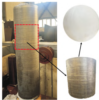
图 13 2024 铝合金铸锭
