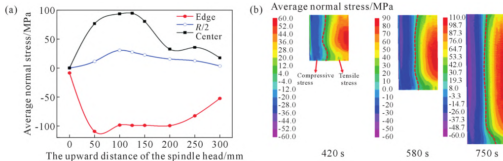
图7 铸造过程中平均主应力分布:(a)同一横截面不同位置主应力值,(b)不同时间纵截面主应力值
