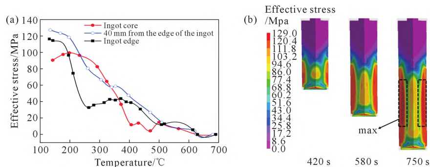
图8 铸造过程中等效应力分布:(a)等效应力随温度变化,(b)等效应力随时间变化
