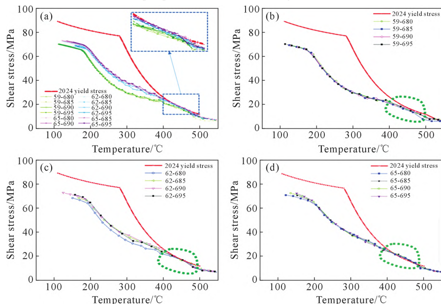
图11 不同工况下切应力分布:(a)剪切应力汇总,(b)59 mm/min,(c)62 mm/min,(d)65 mm/min Fig.11 Shear stress distribution under different working conditions: (a) summary of the shear stress, (b) 59 mm/min, (c) 62 mm/min, (d) 65 mm/min
