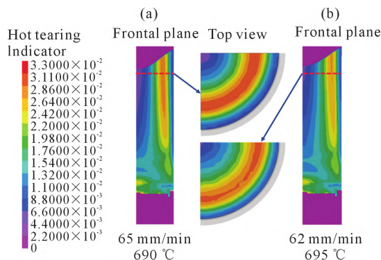
图 12 热裂纹敏感性判断图:(a) 原工况下 HTI 判据图, (b) 优化后 HTI 判据图
