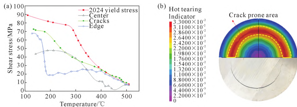
图9 热裂纹敏感性判据图:(a)剪切应力随时间变化,(b)裂纹倾向性模拟结果与铸锭环状裂纹对比
