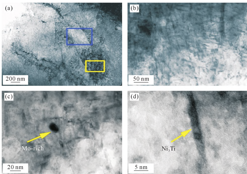
图6 Co-5试样的析出相TEM表征结果:(a)马氏体板条低倍形貌,(b) \text{Ni}_3\text{Ti} 低倍形貌,(c)富Mo相高倍形貌,(d) \text{Ni}_3\text{Ti} 相高分辨图
