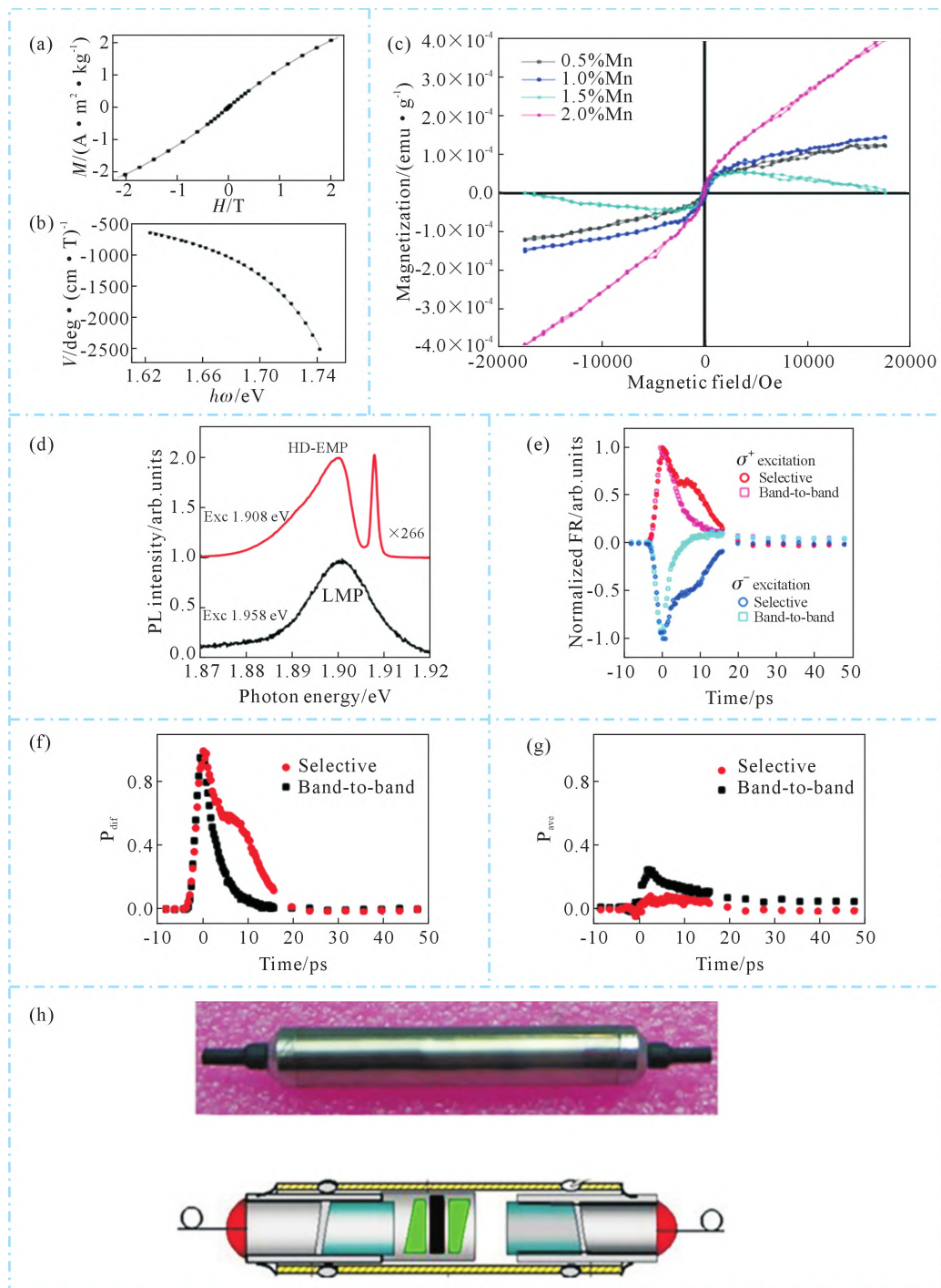
图 8 法拉第磁性器件的相关性能:(a) 2 K 时 \text{Cd}_{0.8}\text{Mn}_{0.2}\text{Te} 的磁化强度随磁场强度的变化曲线,(b) 300 K 下 \text{Cd}_{0.8}\text{Mn}_{0.2}\text{Te} 晶体 Verdet 常数与光子能量的关系,(c) 使用 VSM 记录的室温 M-H 环,用于掺杂 0.5%、1.0%、1.5% 和 2.0% 锰的 \text{CdTe} 纳米颗粒,(d) 在 1.908 和 1.958 eV 的光子能量下激发的 PL 光谱,分别对应选择性激发和带对带激发,(e) 在与 (d) 中相同的激励条件下,使用 \sigma^+ 和 \sigma^- 激励的光感应 FR 信号,(f-g) 频带间激励的 FR 信号的分量及平均分量,(h) 由 \text{Cd}_{0.9}\text{Mn}_{0.1}\text{Te}:\text{V} 单晶制作的磁光隔离器的产品照片和示意图 [93,96,101,105]
