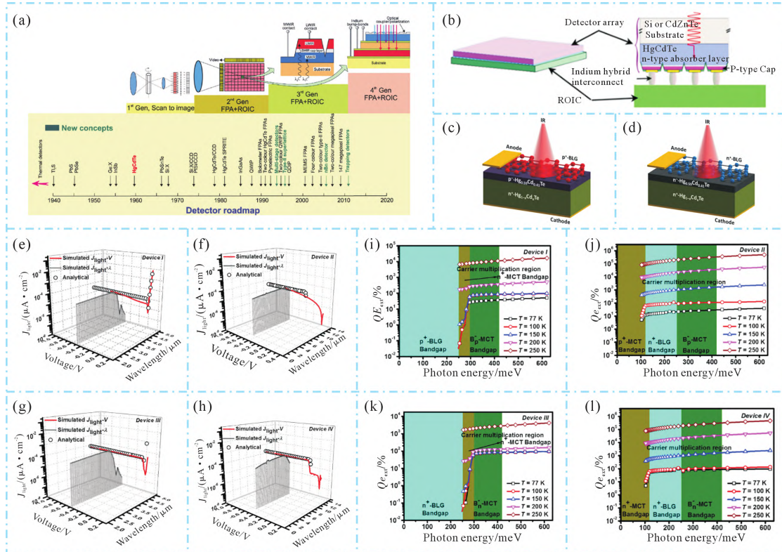
图 10 红外探测器的相关性能:(a) 红外探测器的发展历史和发展路线,(b) HgCdTe/Si 制备 RVS' FPAs 的结构,(c) 红外探测器 p^+-BLG/p-Hg_{0.59}Cd_{0.41}Te/n^+-Hg_{1-x}Cd_xTe ( p^+-p-n^+ ),(d) 红外探测器 n^+-BLG/n-Hg_{0.59}Cd_{0.41}Te/n^+-Hg_{1-x}Cd_xTe ( n^+-n-n^+ ),(e-h) 在 77 K、 50 \mu W/cm^2 的光照强度下装置 I, II, III 和 IV 的 J_{light}-V 和 J_{light}-\lambda 特性,(i-l) 在 -0.5 V 、 50 \mu W/cm^2 的红外照明强度下装置 I, II, III 和 IV 的作为不同温度下入射光子能量的函数模拟 Q_{ext} [118,120,122]
