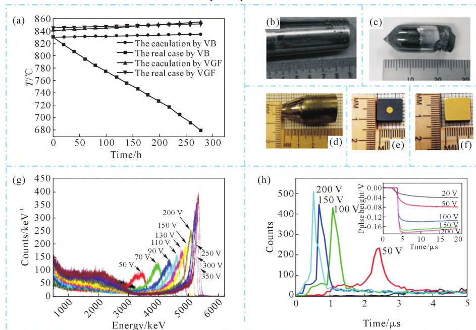
图3 CTS和CZTS晶体及其性能:(a)VB法以及VGF法下Cd源处温度模拟仿真结果与实际对比,(b)生长态的CTS晶锭,(c)通过Cd溶液生长的所得CdTe 0.5 Se 0.5 晶锭,(d)生长的Cd 0.9 Zn 0.1 Te 0.97 Se 0.03 晶锭,(e)11.0×11.0×3.0 mm 3 抛光晶圆小像素,(f)平面探测器,(g)用于发射5486 keV α粒子的 241 Am放射性同位素源照射平面配置的Cd 0.9 Zn 0.1 Te 0.97 Se 0.03 探测器在不同偏置电压下获得的脉冲高度光谱,(h)在相同的实验配置下,从前置放大器脉冲获得的上升时间谱,插图显示了在4个不同的偏置电压下随机选择的典型电荷脉冲 [7,26,31,45]
