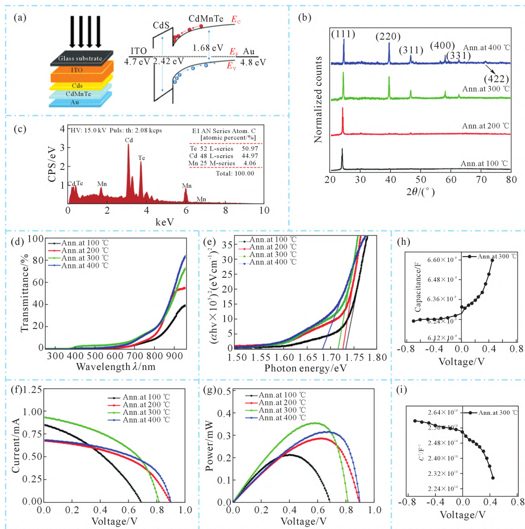
图9 太阳能电池的相关性能:(a) CMT 太阳能电池的器件结构和能带隙图,(b) 在不同退火温度下处理的 CMT 薄膜的 XRD 图谱,(c) 在 300℃ 温度下处理的薄膜的 EDAX 光谱,(d~e) 在不同温度下处理的 CMT 层的透射光谱及相应的 Tauc 图,(f~h) 在不同退火温度下处理的 CMT 太阳能电池的光 I - V 、 P - V 、 C - V 特性,(i) 在 300℃ 下退火的器件的莫特-肖特基图 [114] Fig.9 Related performance of solar cells: (a) device architecture of CMT solar cells and energy band gap diagram, (b) XRD patterns of CMT films processed at different annealing temperatures, (c) EDAX spectra of film treated at 300 °C, (d~e) transmittance spectra and corresponding Tauc graphs of thin CMT layers treated at different temperatures, (f~h) light I - V , P - V and C - V characteristics of CMT solar cells treated at different annealing temperatures, (i) Mott-Schottky plot of the champion device annealed at 300 °C [114]
