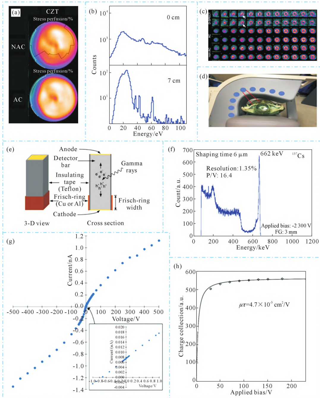
图7 室温辐射探测器在医学中的应用及其性能:(a) 多针 CZT 相机检查一名患者的 NAC 和 AC 牛眼图,图像显示了 NAC 图像中用实线标记的衰减伪影的阈值,(b) CdZnTe 获得的介入手术的能谱,(c) 静息和应力 D-SPECT 图像上偶尔可见的远端下壁衰减伪影(摄取减少,箭头)示例,(d) 排列在龙门架内部的摄像头的鸟瞰图,红线为 9 个探测器的以心脏为中心的视野,(e) 虚拟 Frisch 网格探测器配置示意图,(f) 室温下从 4.8 \times 4.9 \times 9.7 \text{ mm}^3 CZTS-Frisch 栅格探测器获得的 ^{137}\text{Cs} 的光谱,(g) CZTS 探测器在制造成 Frisch 栅格几何形状之前的 I - V 图,(h) ^{241}\text{Am} 的 59.6 keV 伽马峰的电荷收集 [84-86,92]
