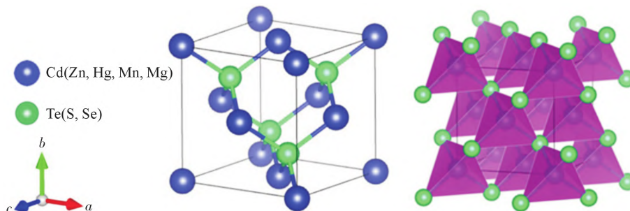
图1 II-VI族多元化合物半导体晶体结构
