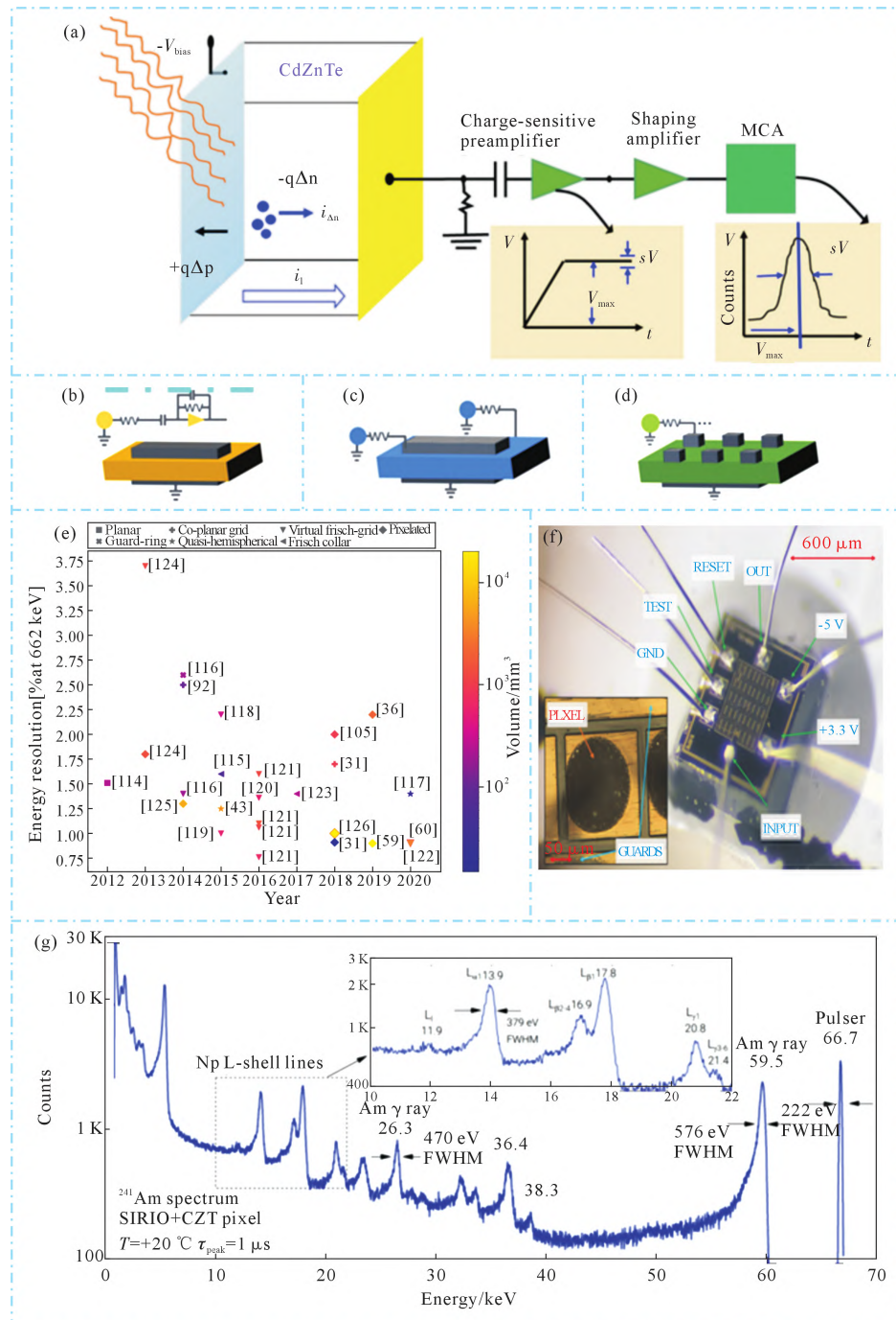
图 6 室温辐射探测器的工作原理、性能及其应用:(a) 标准 CZT 辐射探测系统的框图,(b) MSM 探测器,(c) 共面栅探测器,(d) 像素阵列探测器,(e) 2012 年至 2020 年间基于 CZT 的室温辐射探测器的能量分辨率,(f) SIRIO 电荷敏感前置放大器( 650\times 600\ \mu\text{m}^2 ) 和焊盘引脚的显微图,(g) 使用 Amptek PX5 DPP 在 1\ \mu\text{s} 的最佳峰值时间获得的 ^{241}\text{Am} 源的最佳室温光谱 [80-81]
