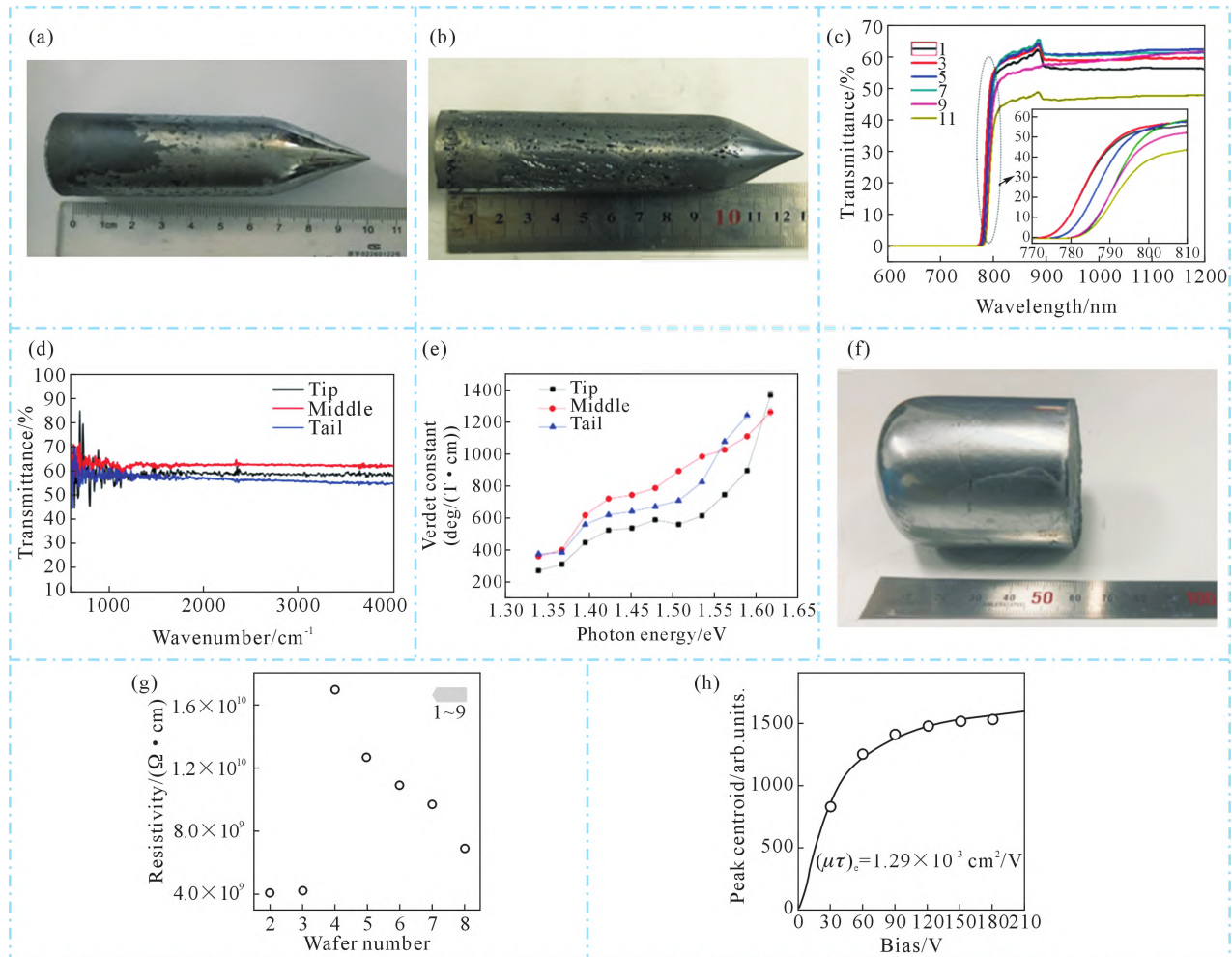
图4 生长态 \text{Cd}_{0.9}\text{Mn}_{0.1}\text{Te}:\text{V} 和 \text{Cd}_{0.95}\text{Mn}_{0.05}\text{Te}_{0.98}\text{Se}_{0.02}:\text{In} 晶锭及其性能:(a) 第一次生长,(b) 第二次生长,(c) 典型的 \text{Cd}_{0.9}\text{Mn}_{0.1}\text{Te}:\text{V} 晶体紫外-可见-近红外透过光谱,(d) 室温下 \text{Cd}_{0.9}\text{Mn}_{0.1}\text{Te}:\text{V} 晶体的红外透过率曲线,(e) 室温下 \text{Cd}_{0.9}\text{Mn}_{0.1}\text{Te}:\text{V} 晶体的费尔德常数与光子能量关系图,(f) 垂直 Bridgman 技术在低压下生长 \text{Cd}_{0.95}\text{Mn}_{0.05}\text{Te}_{0.98}\text{Se}_{0.02}:\text{In} 晶锭,(g) 从 CMTS 晶锭上切下的晶片的电阻率,(h) 59.5 keV 伽马射线的峰值质心与偏压的关系图 [47,56]
