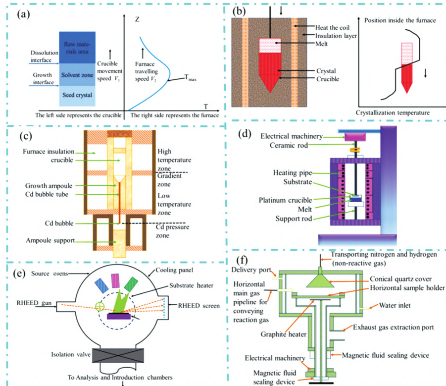
图2 不同晶体生长方法示意图:(a)移动加热器法原理图,(b)垂直布里奇曼法,(c)垂直梯度凝固法,(d)液相外延法,(e)分子束外延法,(f)金属有机化学气相沉积法 [21-24]
