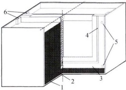
1- 外模;2- 镓铜合金;3- 内模;4- 密封条;5- 紧固螺栓;6- 定位卡槽
