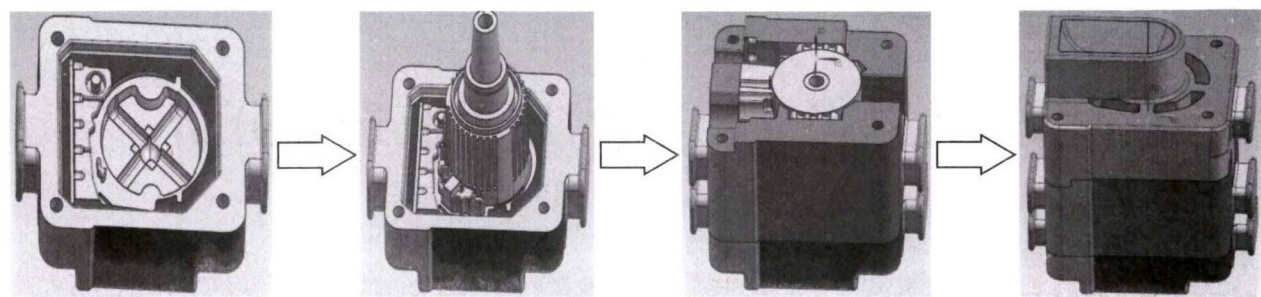
图 7 砂型分型工艺 Fig.7 Parting process of sand mould
