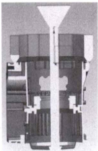
图 6 增加冷铁 Fig.6 Adding the chiller
