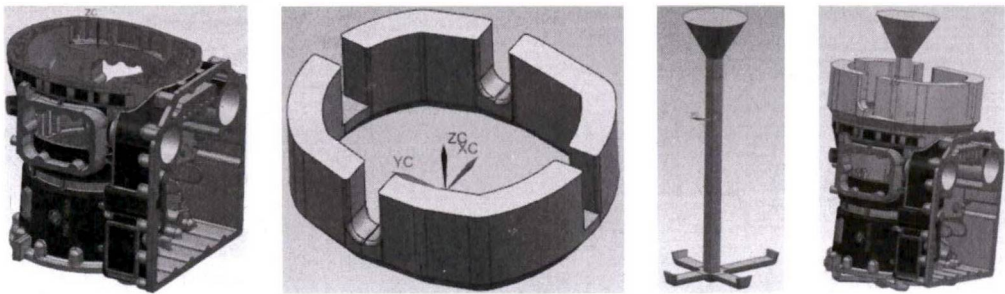
图 4 三维浇注系统 Fig.4 3D drawing of pouring system
