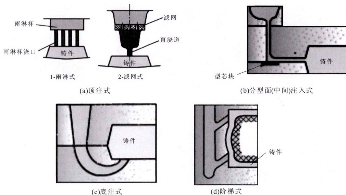
图2 不同浇注方式 Fig.2 Different pouring methods
